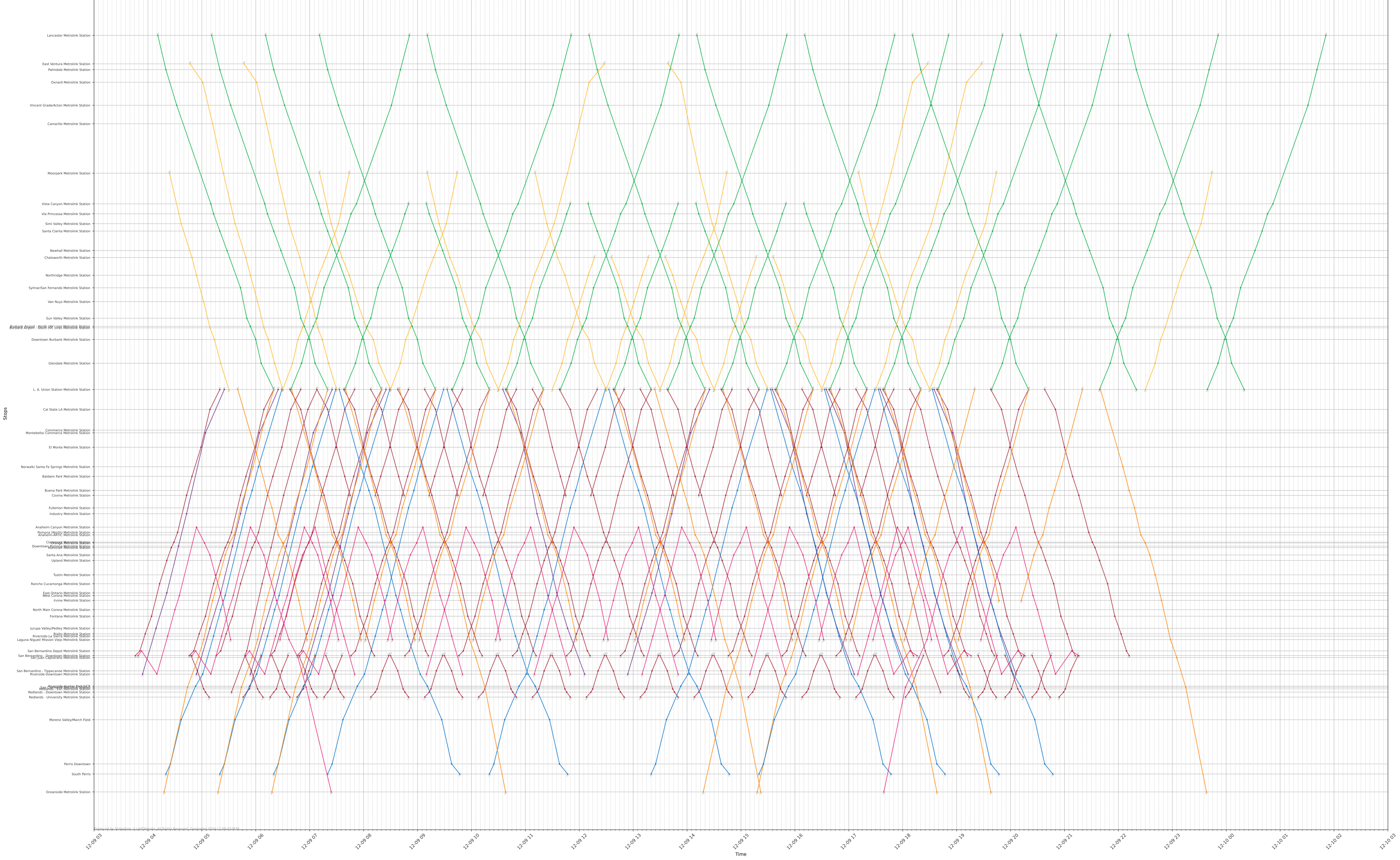
LA Metrolink - Systemwide Stringline (3x) Stringline
